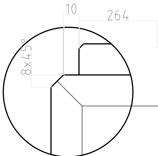
Detaliu A scara 5:1
